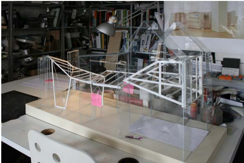
Maqueta. Paso peatonal en Tourcoing. Atelier 9.81, 2011.
