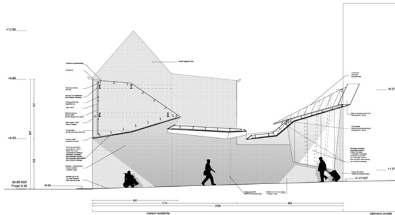
Sección. Paso peatonal en Tourcoing. Atelier 9.81, 2011.
